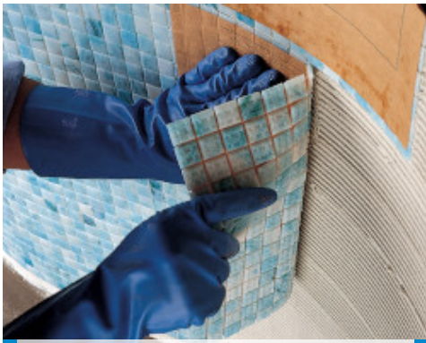
Assentamento de pastilha de vidro 2x2 em piscina com Adesilex P10 mais Isolastíc diluído 1:1 com água
